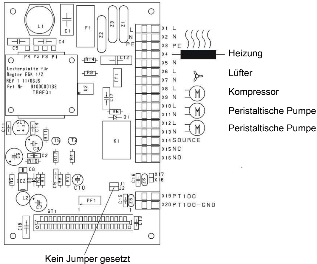
Abb. 3: A100042 Netz- und Regelplatine
