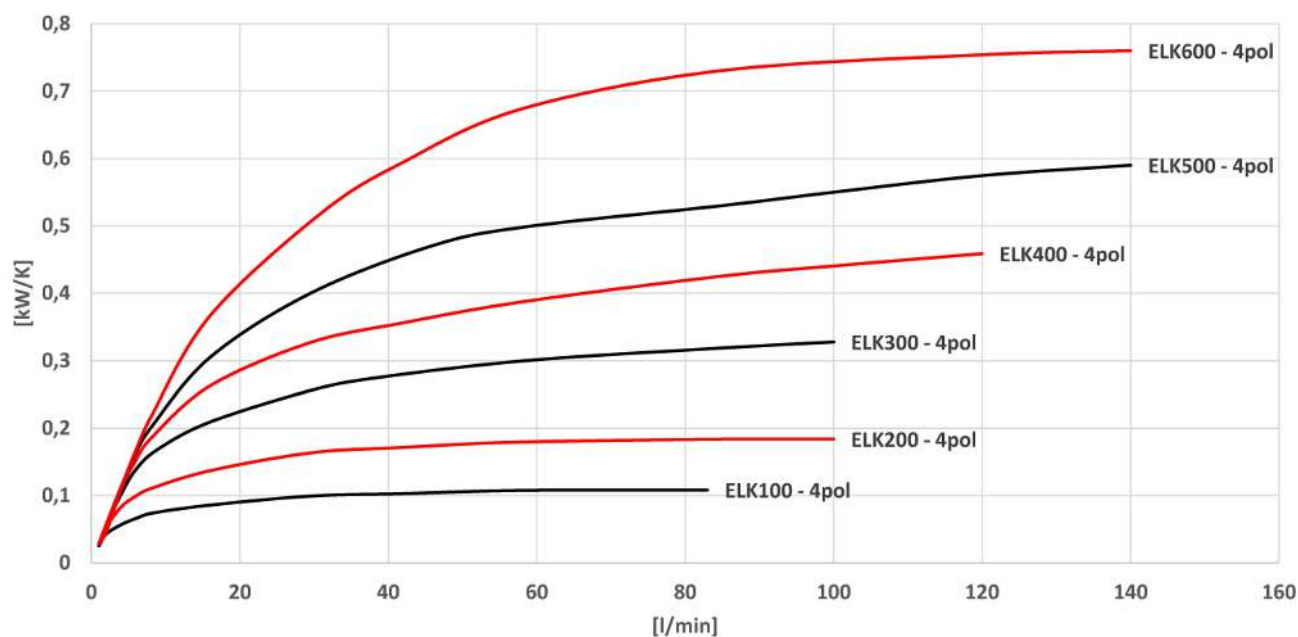
Il. 2: Potencia específica de refrigeración:
