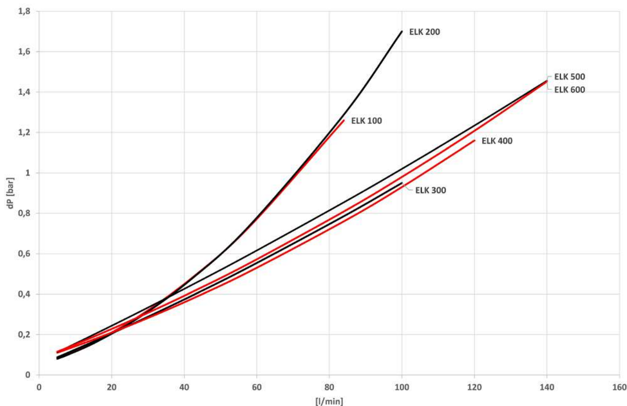
Il. 3: Pérdida de presión
