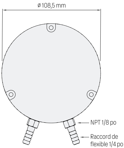
Figure 15 Dimensions de la protection de refroidissement
