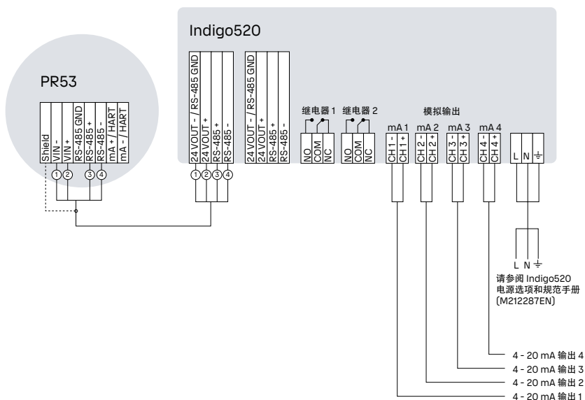
图 46 PR53 和 Indigo520 的接线图
