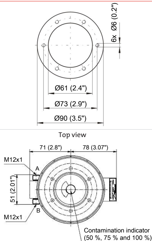
Flange pattern as per DIN 24557 Part 2
