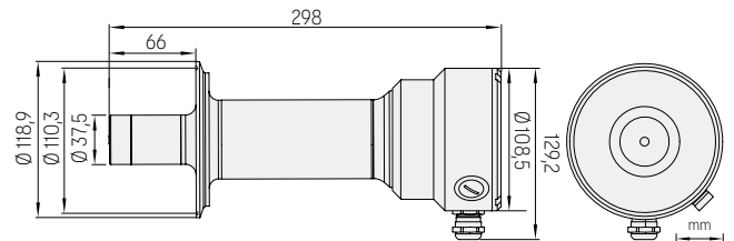
Abmessungen der PR53AP 4"-Sanitary-Dichtung, Tiefe 66 mm
