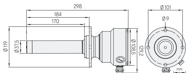
Abmessungen des PR53APEX Tankbodenflansches, Tiefe 170 mm
