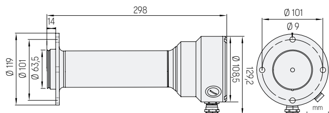
Abmessungen des PR53APEX Tankbodenflansches, Unterputzmontage
