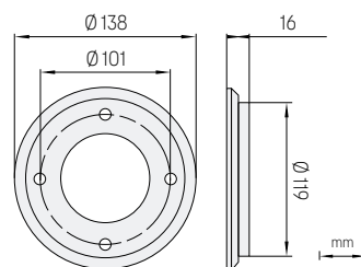
Abmessungen des PR53APEX Tankboden-Schweißflansches
