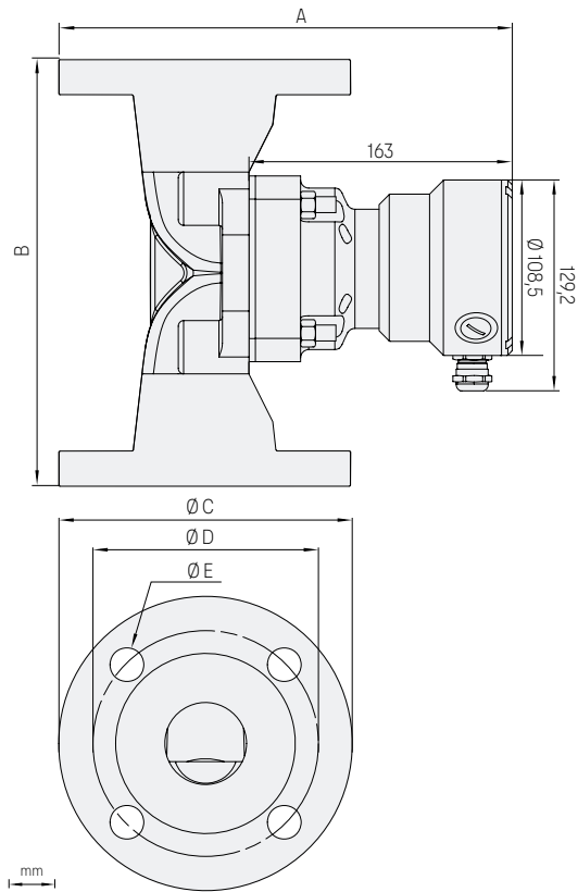
Abmessungen des PR53WEX Ventilgehäuses
