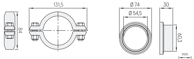
Abmessungen der PR53GCEX Schelle für Sandvik Coupling L
