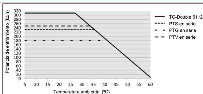
Modelo TC-Double 6112 (X2)
