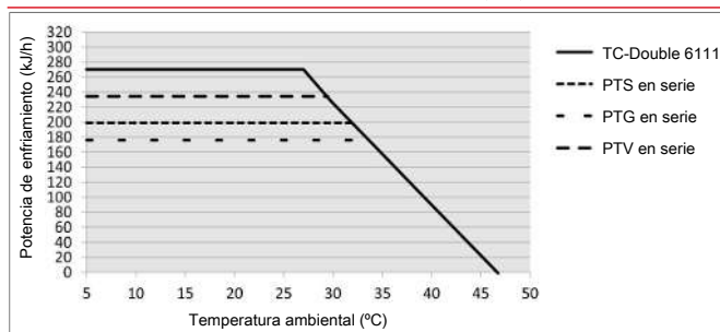
Modelo TC-Double 6111 (X2)
