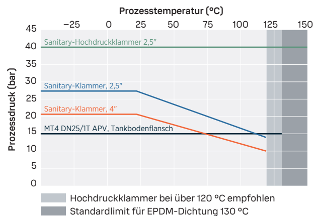
PR53AP Prozessdruck
