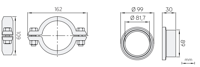
Abmessungen des PR53GP, Schelle für Sandvik Coupling L
