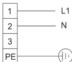
Сетевое подключение
