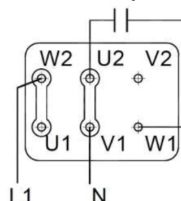
Moteurs à courant alternatif avec condensateur d'exploitation
