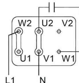
Motor de corriente alterna con condensador de funcionamiento
