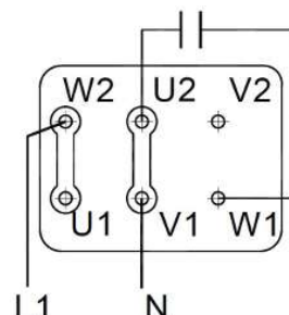
Moteurs à courant alternatif avec condensateur d'exploitation
