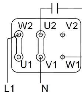
двигатель переменного тока с рабочим конденсатором
