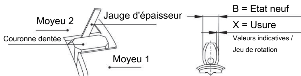
Fig. 3: Embrayage pompe à gaz à mesurer
