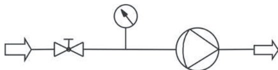
Fig. 2: Contrôle du joint à soufflet
