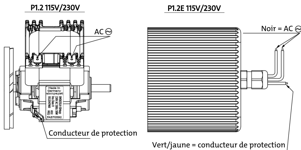
Fig. 2: Raccordements électriques de pompes P1.2
