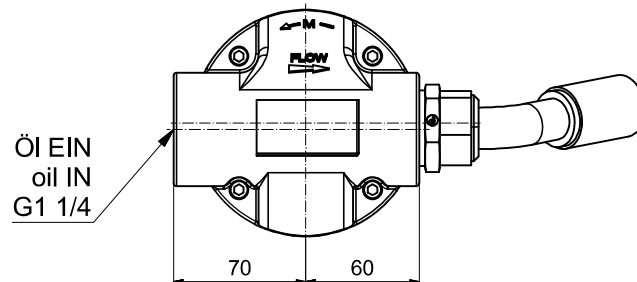
Ansicht A
