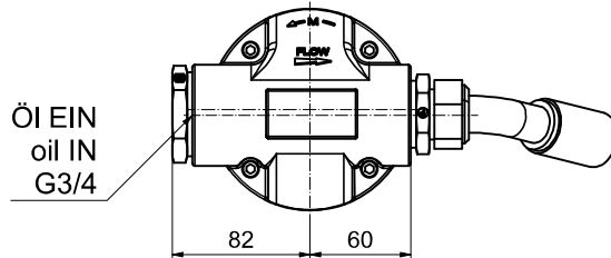
Ansicht A
