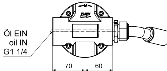
Ansicht A
