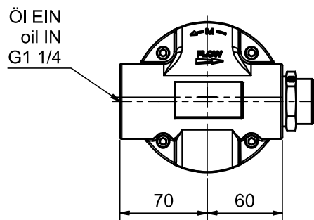
Ansicht/view A ( 1 : 3 )
