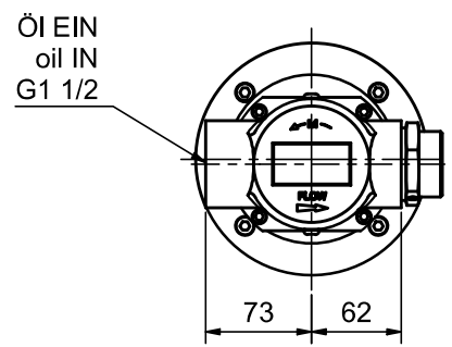
Ansicht/view A ( 1 : 4 )
