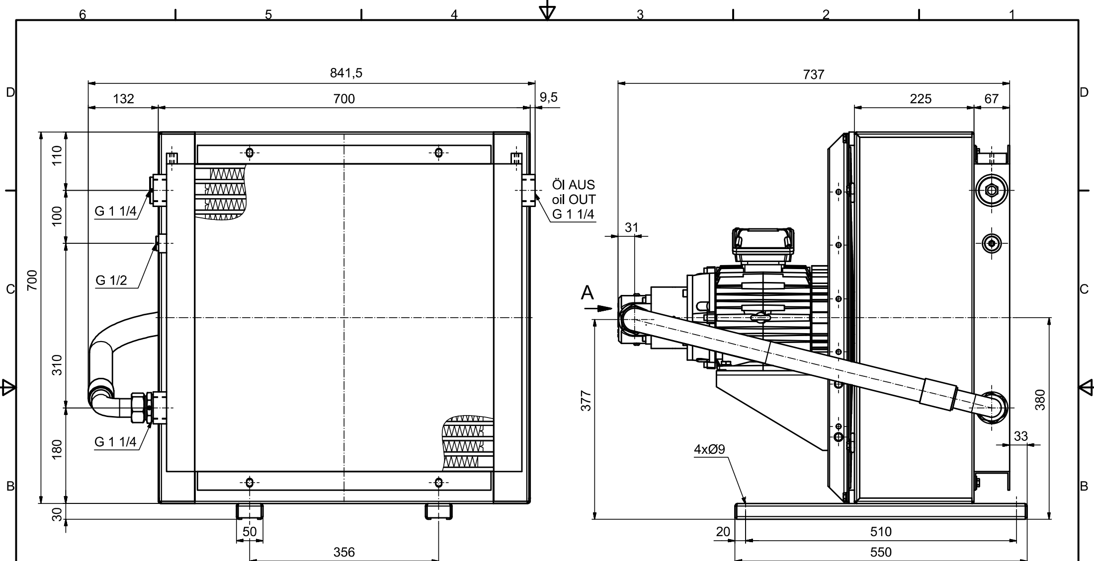
Ansicht A
