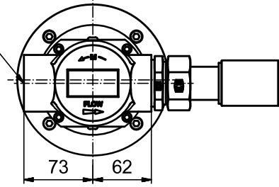
Ansicht A
