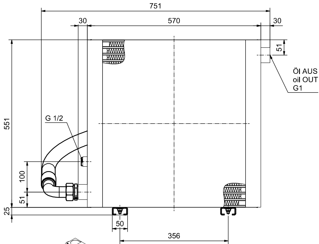
Ansicht/view A ( 1 : 4 )
