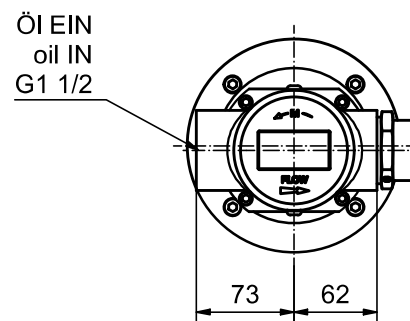
Ansicht/view A ( 1 : 4 )
