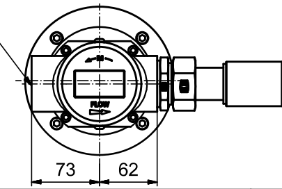
Ansicht A
