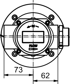
Ansicht/view A ( 1 : 4 )
